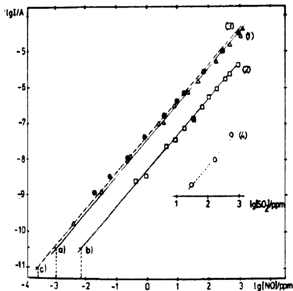
Abb. 2. Eichkurven für den Nachweis von NO in N 2 und in Luft in doppeltlogarithmischer Auftragung. (1) NO in N 2 durch Fluoreszenz; Nachweisgrenze a). (2) NO in Luft durch Fluoreszenz; Nachweisgrenze b). (3) NO in N 2 und Luft durch Chemilumineszenz; Nachweisgrenze c). — Zur Bestimmung der Querempfindlichkeit von SO 2 zeigt Kurve (4) die Abhängigkeit der SO 2 -Fluoreszenzintensität vom SO 2 -Gehalt der Luft, wie sie mit dem Fluoreszenzgerät gemessen wurde. Von allen Werten wurde jeweils das Untergrundsignal subtrahiert. Für die Fluoreszenzmessungen betragen der Gesamtdruck 35 Torr und die Zeitkonstante 10 s, für die Chemilumineszenzmessungen betragen der Gesamtdruck 4 Torr und die Zeitkonstante 1 s.
