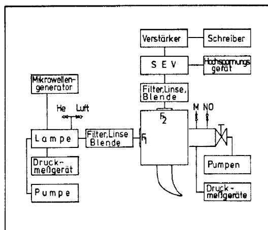
Abb. 1. Blockdiagramm der Fluoreszenzanordnung. F 1 und F 2 bezeichnen die Quarzfenster, M den Einlaß für Zusatzgase.
