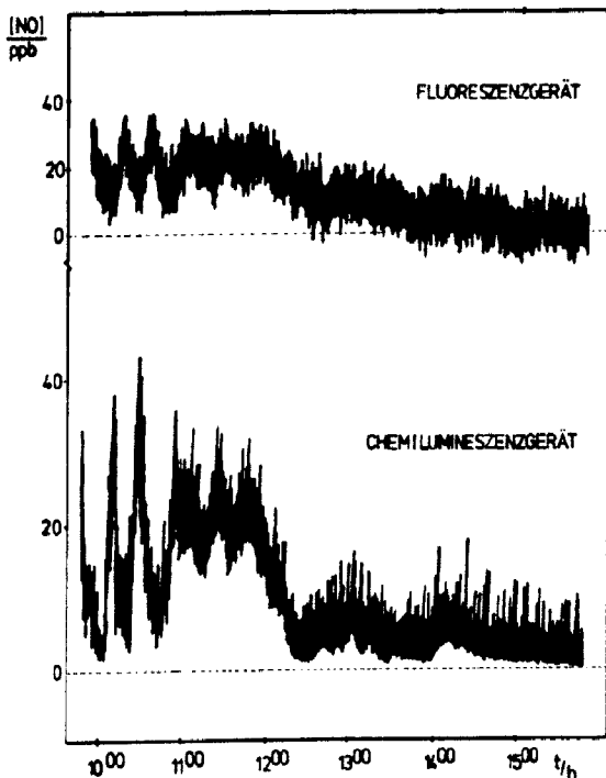
Abb. 3. Luftmessung mit Fluoreszenz- und Chemilumineszenzgerät. — Ausschnitt aus einem Tagesverlauf der NO-Konzentration in der Luft vom 27. 11. 1975 an der Ruhr-Universität Bochum, Gebäude NC, 10. Stockwerk, Westseite. — Fluoreszenzgerät: Gesamtdruck 35 Torr; Zeitkonstante 10 s. Chemilumineszenzgerät: Gesamtdruck 4 Torr; Zeitkonstante 1 s.
