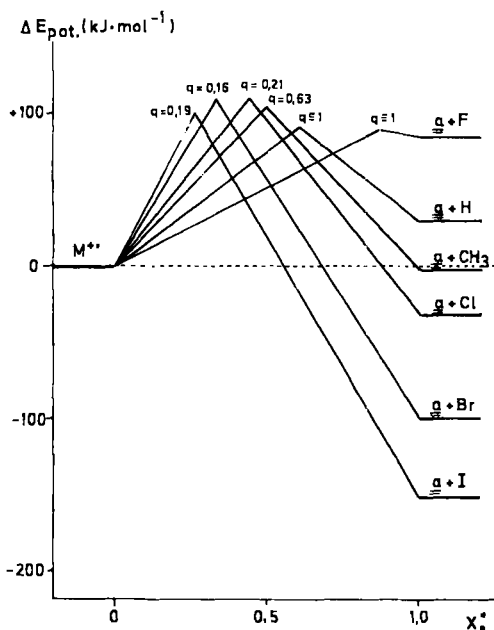
Abb. 3. Hammond-Diagramm der intramolekularen Substitution in den Molekül-Ionen 1a–1g ( X_{\ddagger}^{\circ} = Position des Übergangszustandes auf der Reaktionskoordinate; q = Energieaufteilungsquotient)
