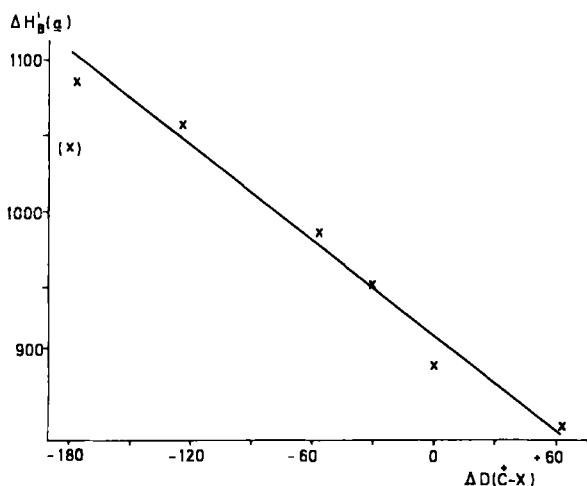
Abb. 2. Abhängigkeit der scheinbaren Bildungsenthalpie \Delta H_B^{\dagger}(\mathbf{a}) von der relativen Dissoziationsenergie \Delta D(\overset{\ddagger}{\text{C}} - \text{X}) der Substituenten in den Molekül-Ionen 1a – 1g
